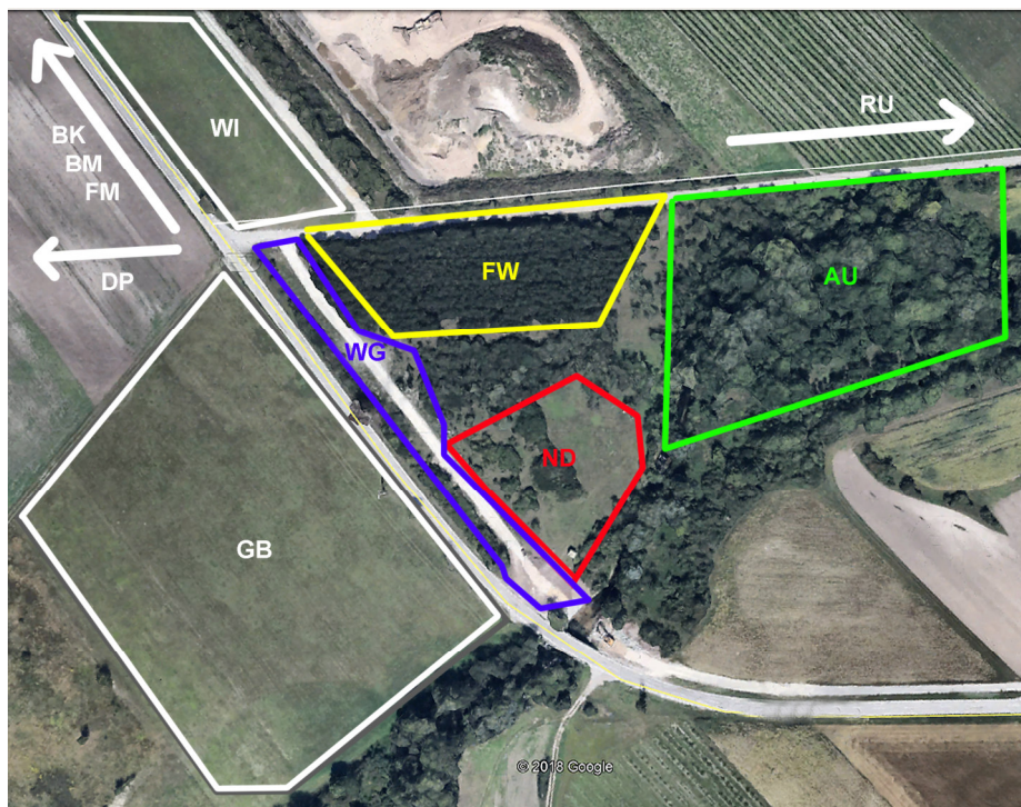
Abb. 1: Lage des Untersuchungsgebietes mit seinen Teilgebieten (farbig) und den näheren zusätzlich bearbeiteten Flächen (weiß). Abkürzungen: siehe Tab. 2 . / Map of the study area with specified sites (in colours) and the nearby additional sites (white). Kartengrundlage: Google Earth.
